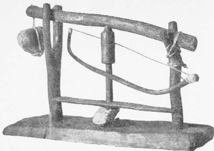
Vyobr. 3. Vrtačka z doby kamenné.
